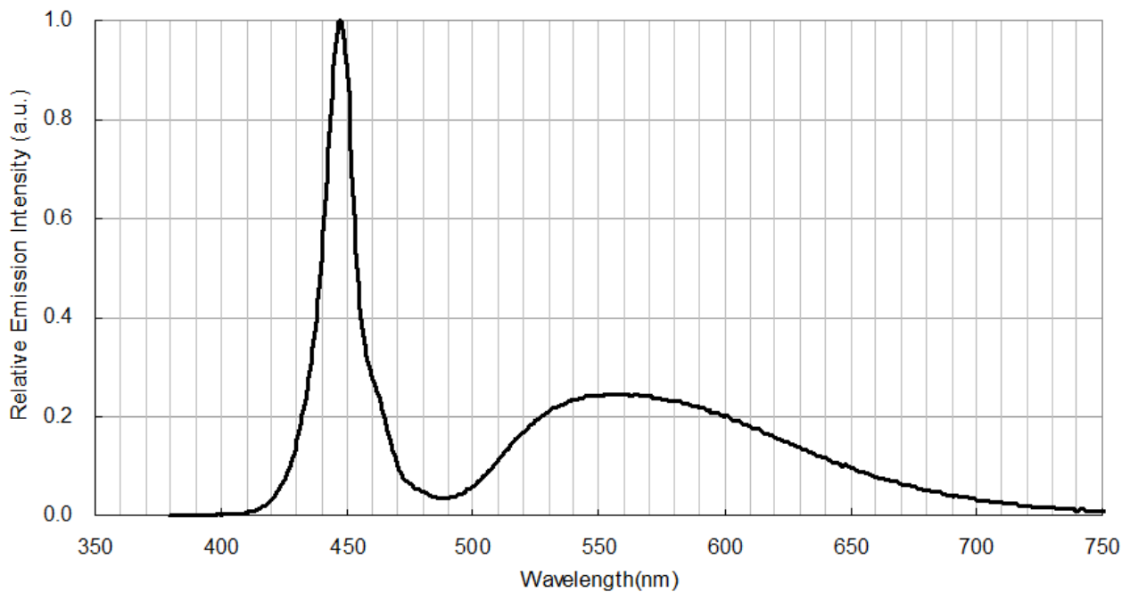
Spectrum( T_A=25^{\circ}\text{C} , I_{FP}=20\text{mA} )
